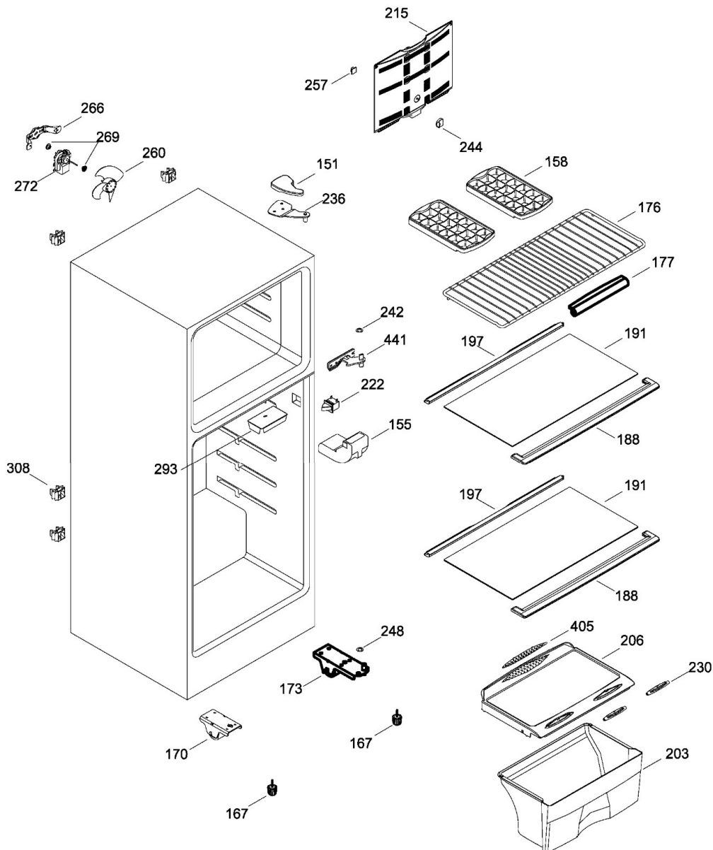
206.- TAPA CAJON LEGUMBRES ENS. VEG PAN ASM.
