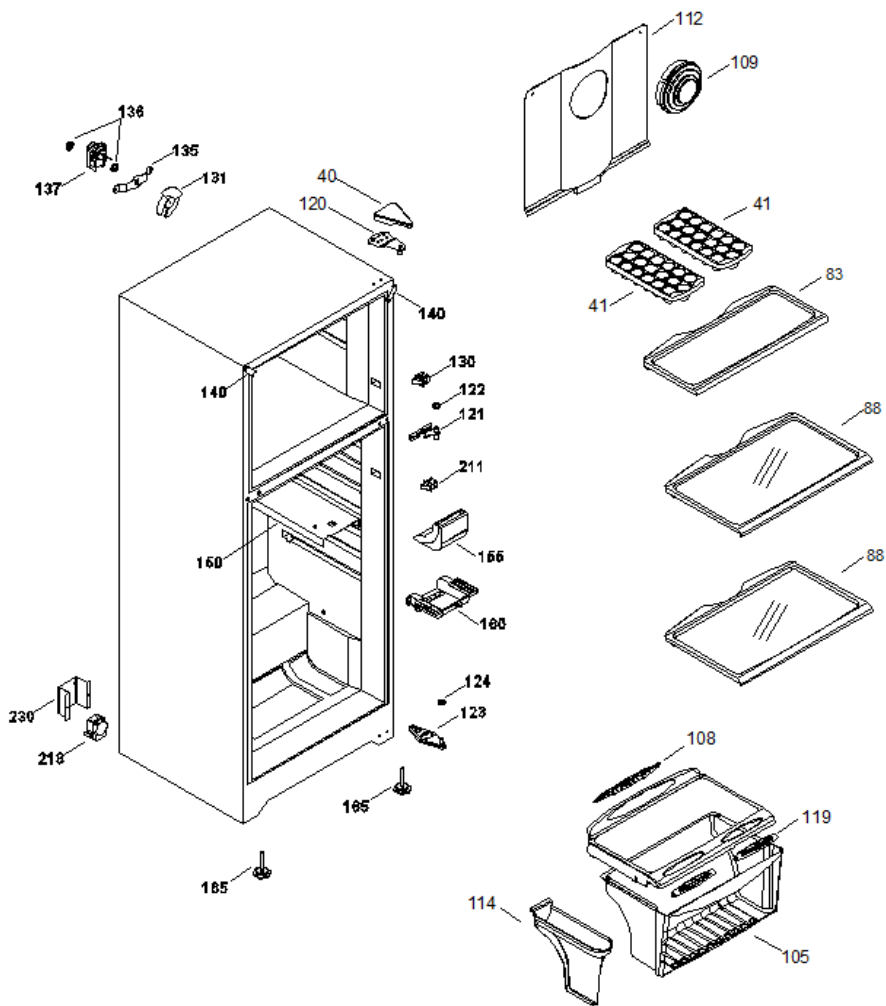
106.- TAPA CAJON LEGUMBRES ENS. VEG PAN ASM.
