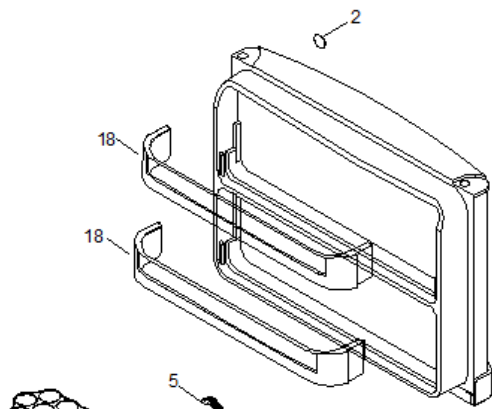
1 PUERTA CONGELADOR ENS. COMPL. DOOR FZ ASM.
