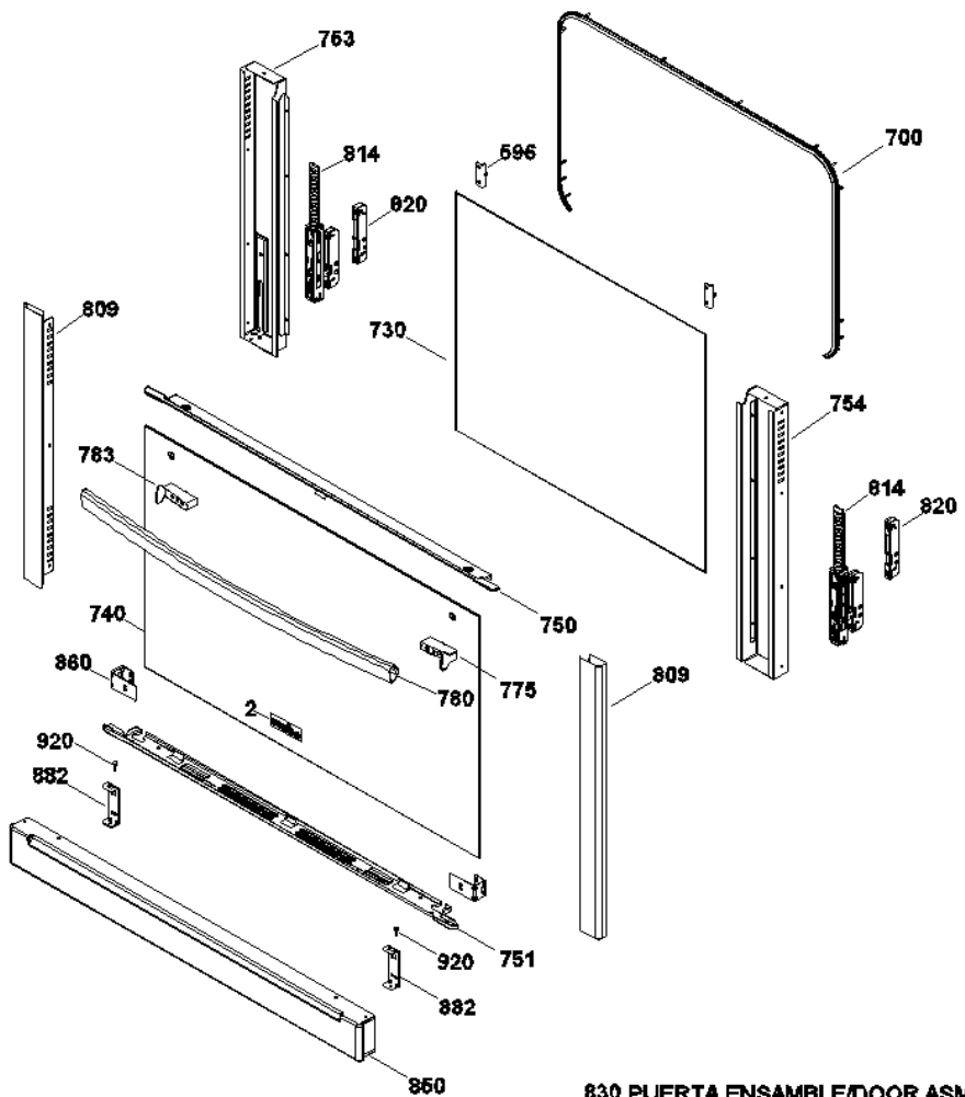
830 PUERTA ENSAMBLE/DOOR ASM
